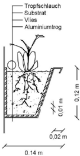
Abb. 32: Schematische Skizze eines Troges des wandgebundenen Systems.
